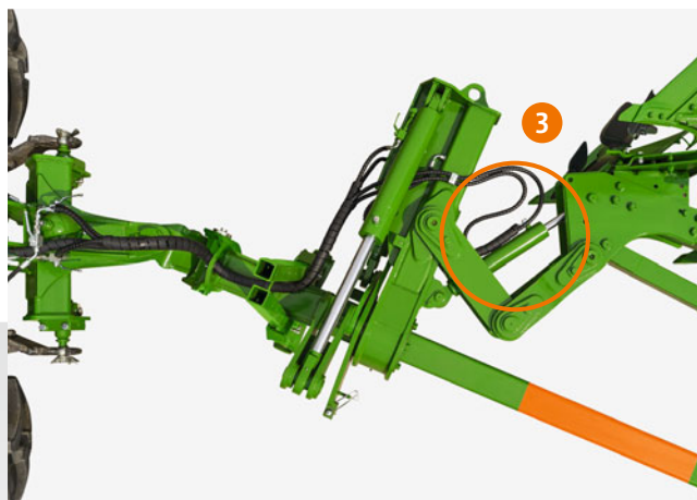
Гидравлическая настройка первой борозды
