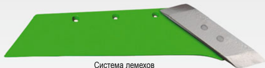
Система лемехов со сменной накладкой
